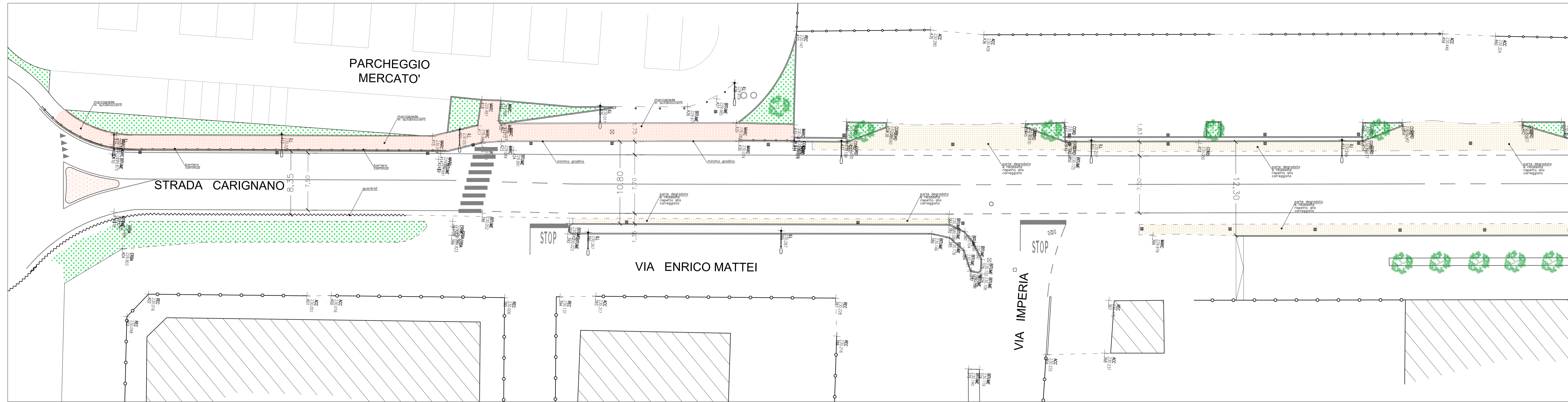
RILIEVO STATO DI FATTO – TRATTO A scala 1:200
